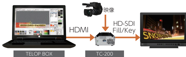
※TELOP BOXにTC-200は含まれません。別途ご用意ください。
